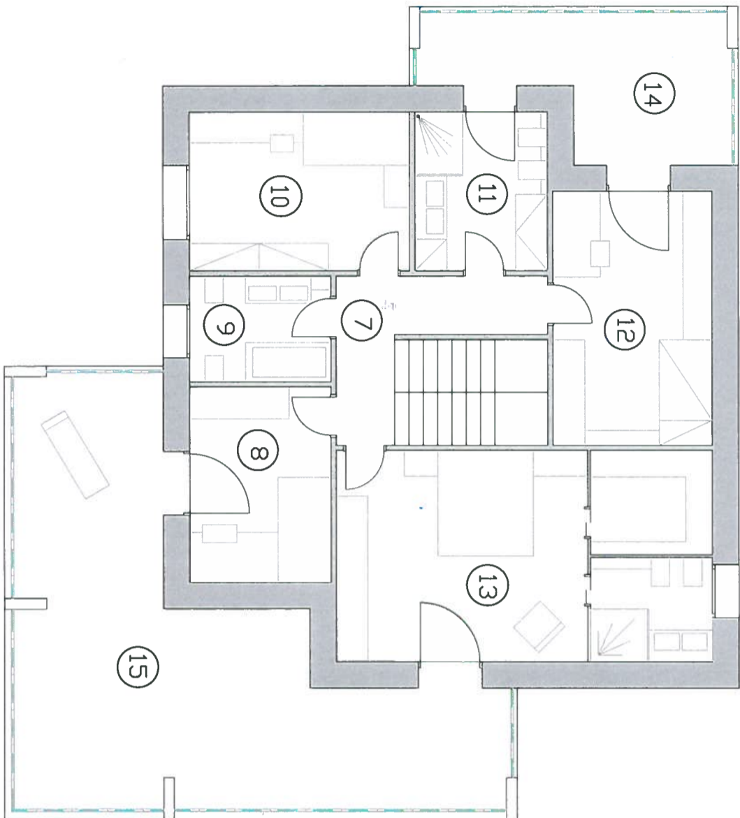
PIANO PRIMO - Scala 1:100
