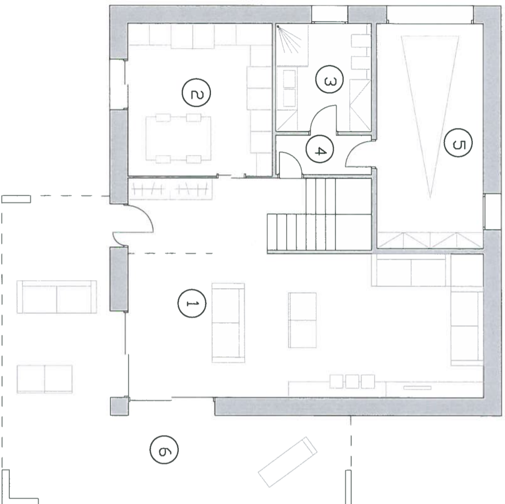
PIANO TERRA - Scala 1:100
