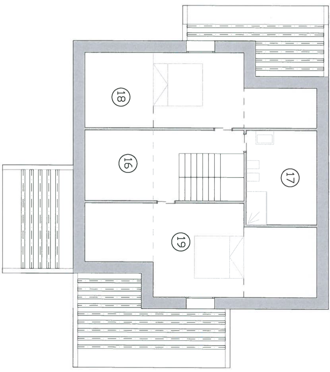
PIANO MANSARDATO - Scala 1:100
