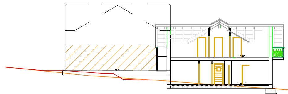
SEZIONE X - Y
